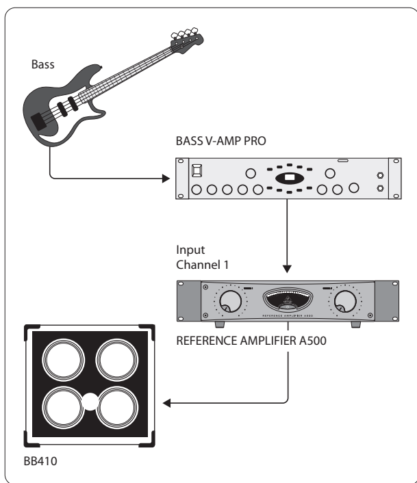
Рис. 3.2: Мостовой режим
