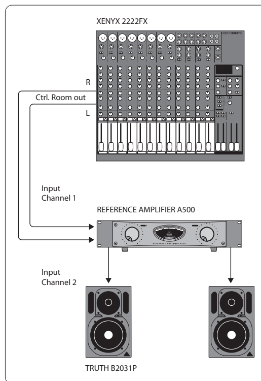
Рис. 3.1: A500 в режиме стерео
