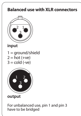
Рис. 4.1: Разъемы XLR
