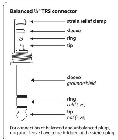
Рис. 4.3: 6,3 мм- стереоштекер
