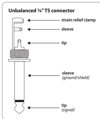
Рис. 4.2: 6,3 мм- монофонический штекер
