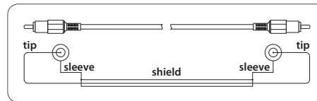
Рис. 4.4 Несимметричное подключение с помощью кабеля с RCA- разъемами
